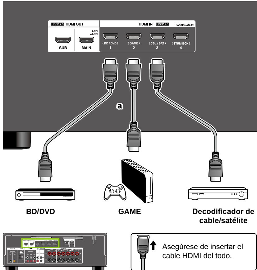
a Cable HDMI
