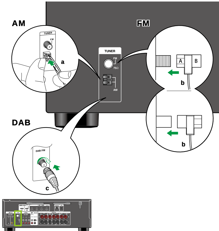
a Antena en bucle AM, b Antena FM para interiores
