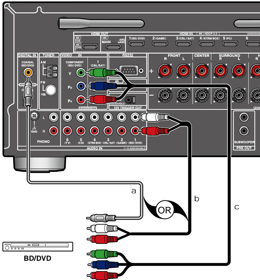
a Cable coaxial digital, b Cable de audio analógico, c Cable de vídeo componente
